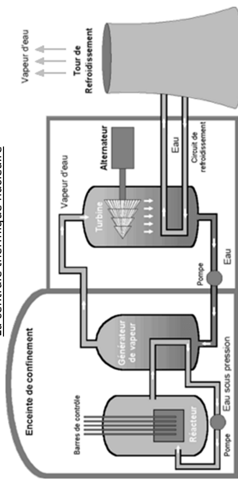
La centrale thermique nucléaire
